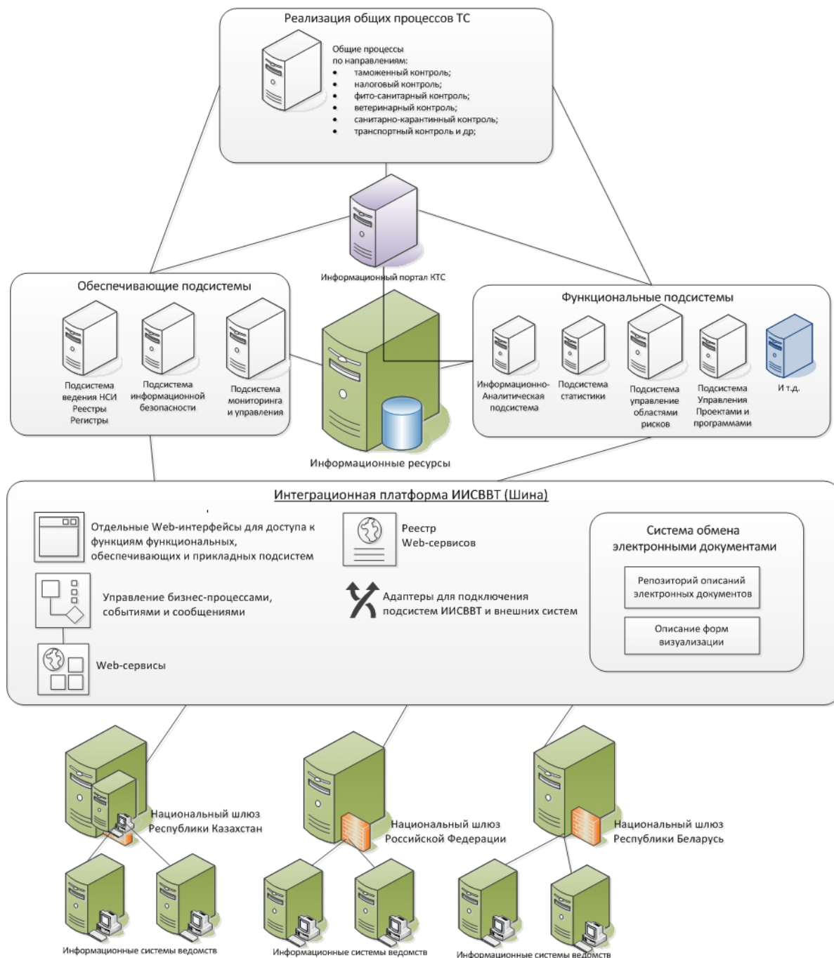
Рис.1 Общая схема ИИСВВТ.
